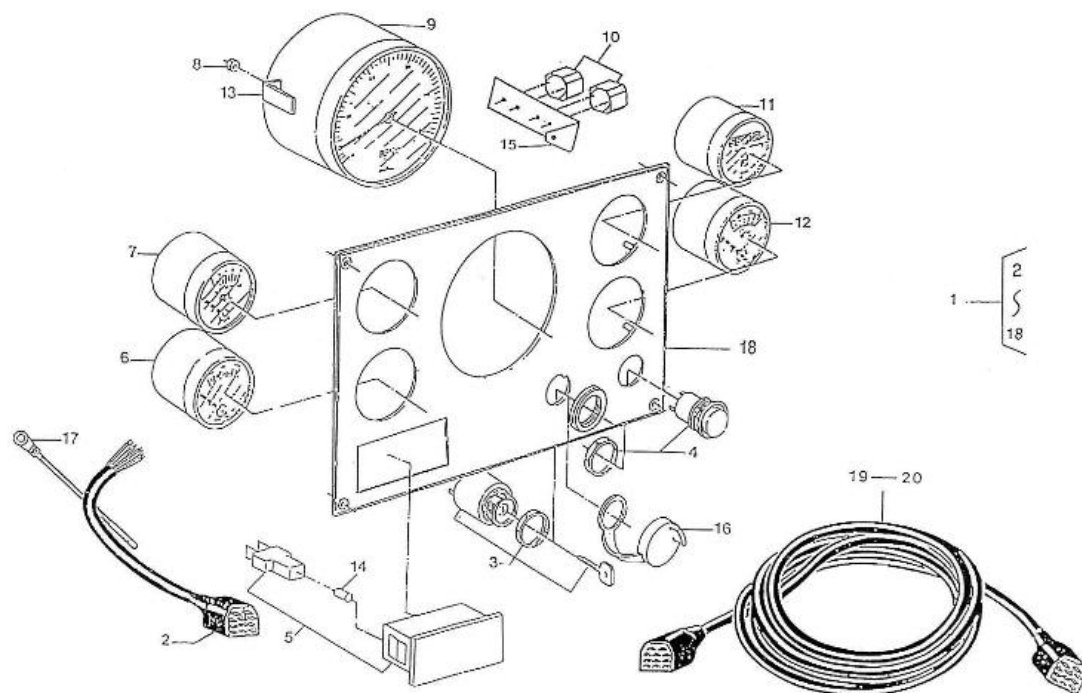
PANEL "C" (Optional équipement)
